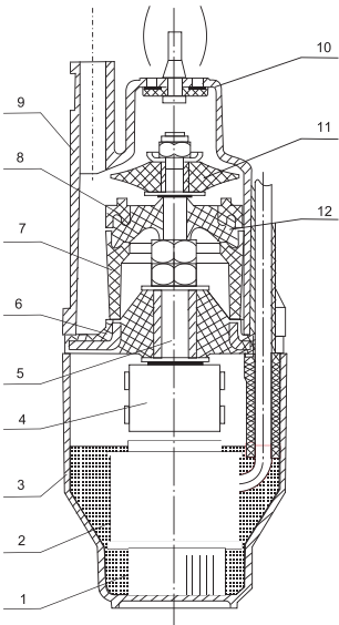
Рис. 1. Устройство насоса
