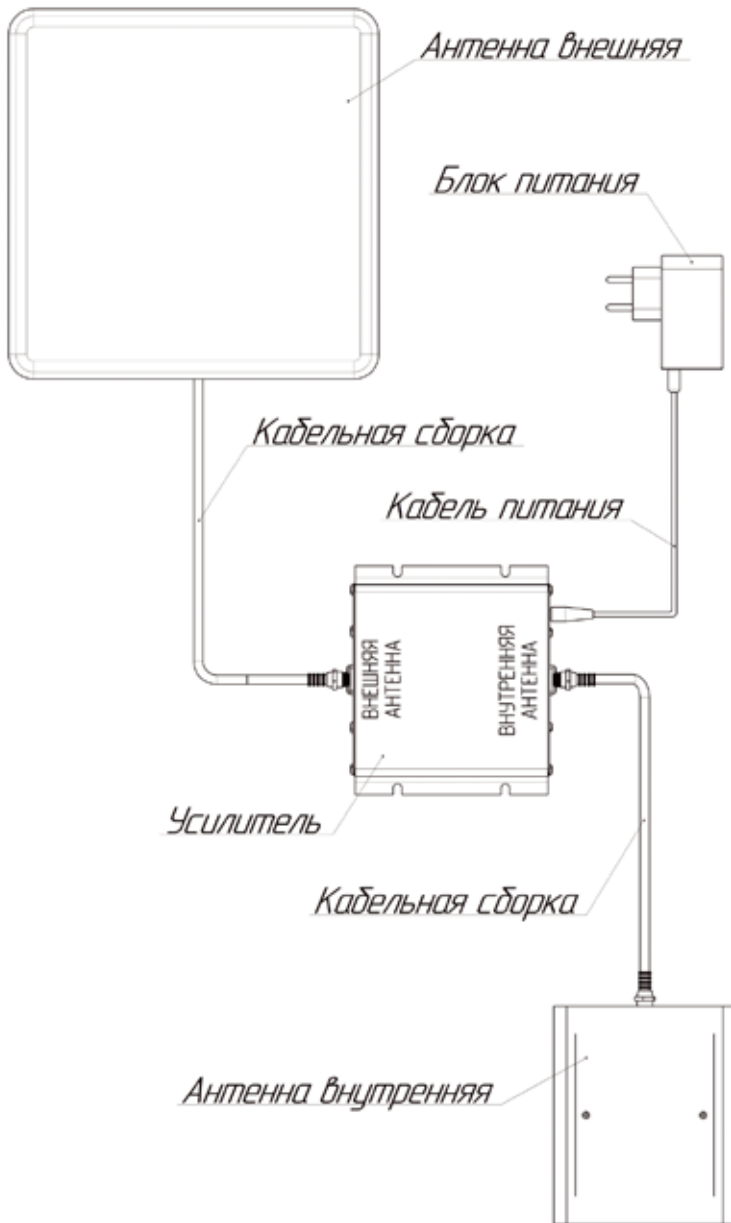
Рисунок 6. Схема подключения
