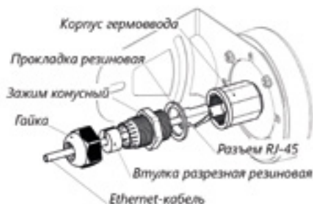
Рис. 2. Подключение Ethernet-кабеля к внешнему блоку
