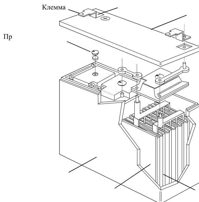
Рис 1. Конструкция моноблоков DELTA серии HR
