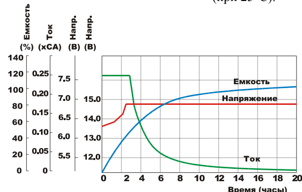
Рис 4. График заряда постоянным напряжением (при 25°C).
