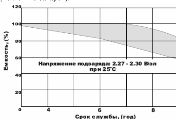
Рис 7.2. Срок службы в буферном режиме работы (10-летние батареи).
