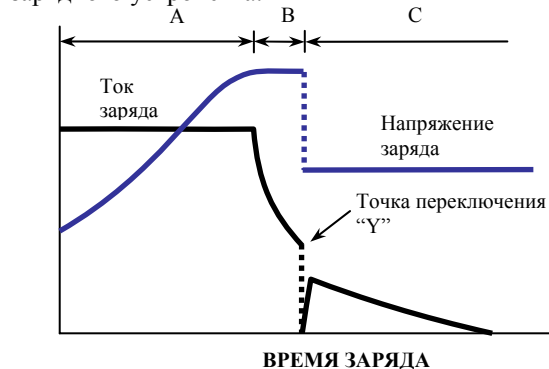
Рис 5. Зарядные характеристики двухстадийного зарядного устройства.
