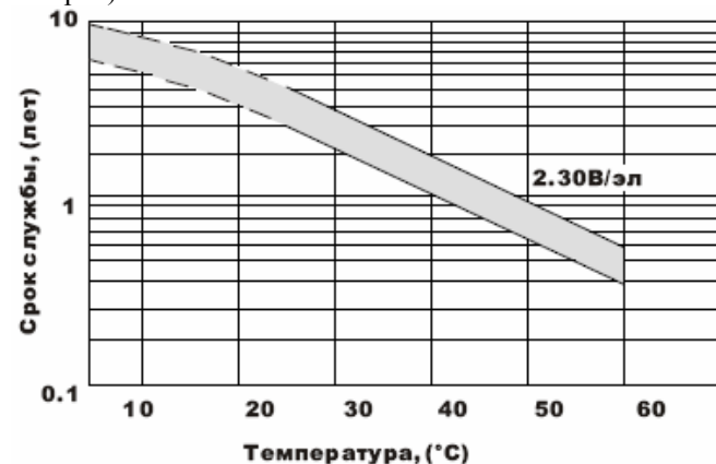
Рис 10.1. Зависимость срока службы в буферном режиме от температуры окружающей среды (5-летние батареи).
