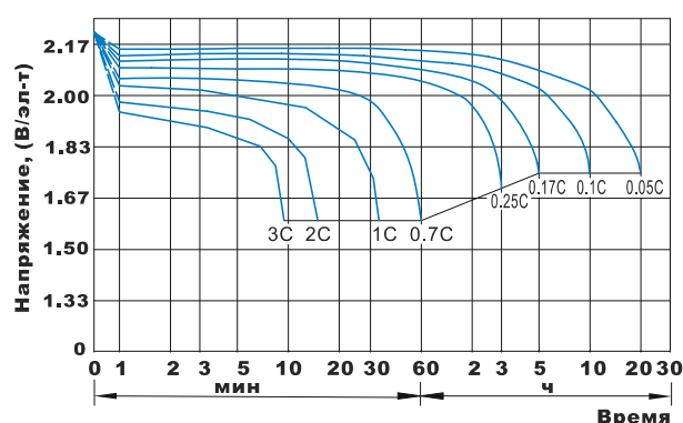
Рис 3. Разрядные кривые постоянным током при 25°C
