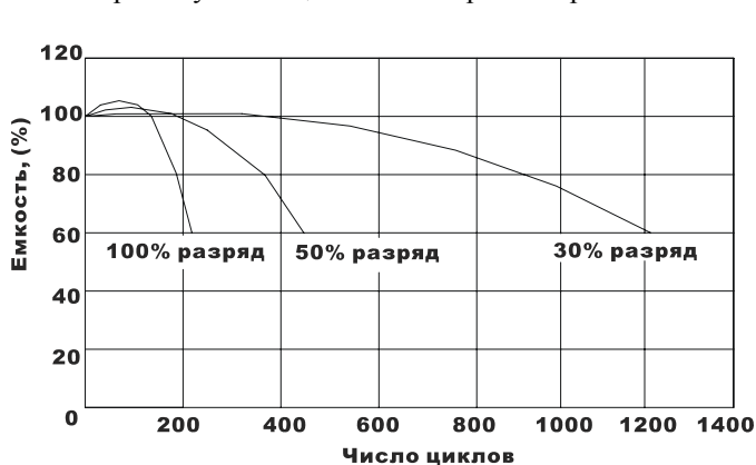
Рис 8. Срок службы в циклическом режиме работы.
