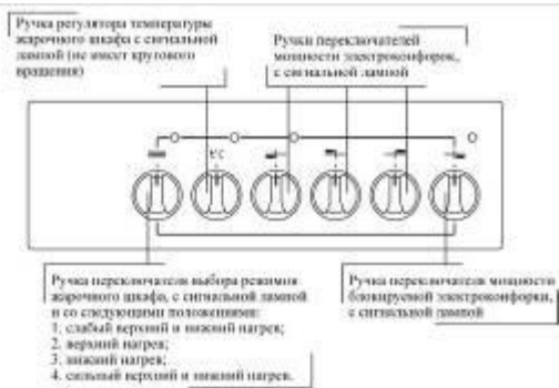
Рис. 10. Передняя панель плиты ЭП411
