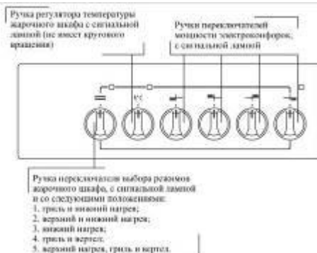
Рис. 9. Передняя панель плиты ЭП403
