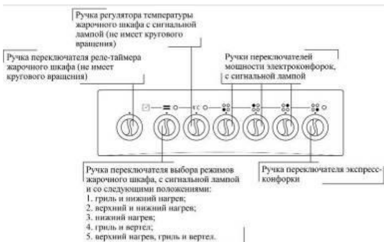
Рис. 14. Передняя панель плиты ЭП4/1эЗр3МС, ЭП4/1эЗр3М2С
