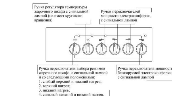
Рис. 9. Передняя панель плиты ЭП 411СТ
