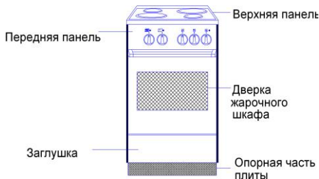
Рис. 6. Электроплита
