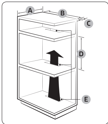
Вбудована шафа (мм)
