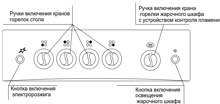
Рис. 12. Передняя панель плиты
