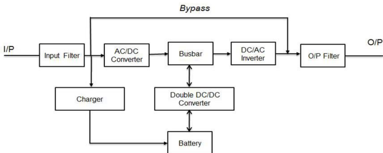
Рис.1 Блок-схема ИБП
