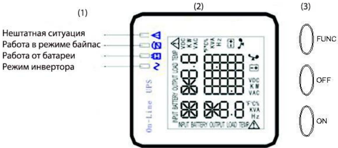
Рис. 4. Панель управления ИБП
