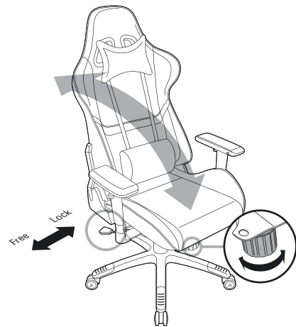
Откидной механизм спинки с возможностью режима качания и блокировки
