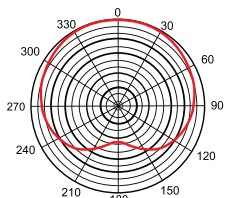
1 кГц кезіндегі бағыттылық диаграммасы
