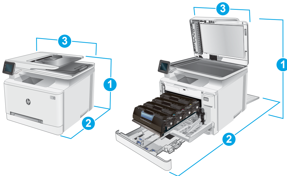
Рисунок 1-2 Размеры моделей cdw, fdn и fdw
