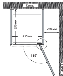
Встроенный монтаж
