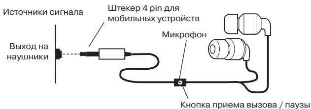
Рис. 1. Схема подключения
