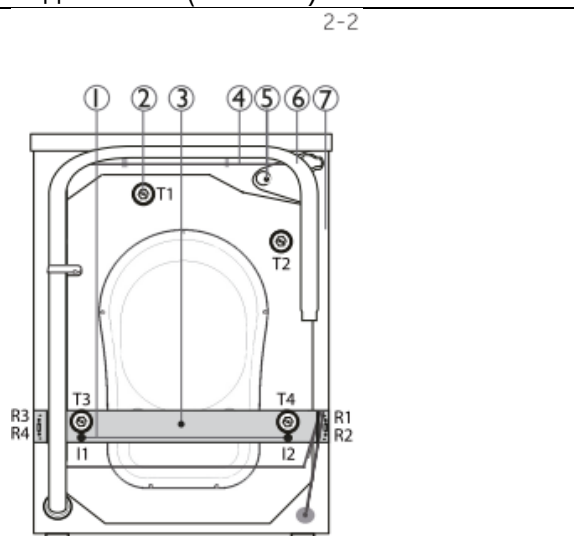
Задня стінка (Мал. 2-2)
