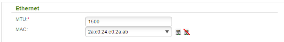
Рисунок 121. Страница добавления соединения типа PPTP + Статический IP. Раздел Ethernet.
