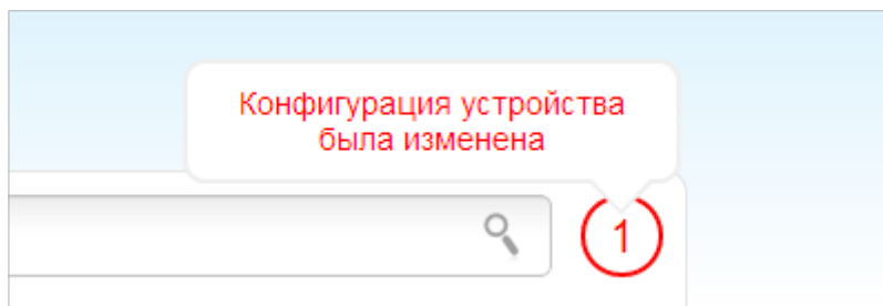
Рисунок 23. Уведомления web-интерфейса.
