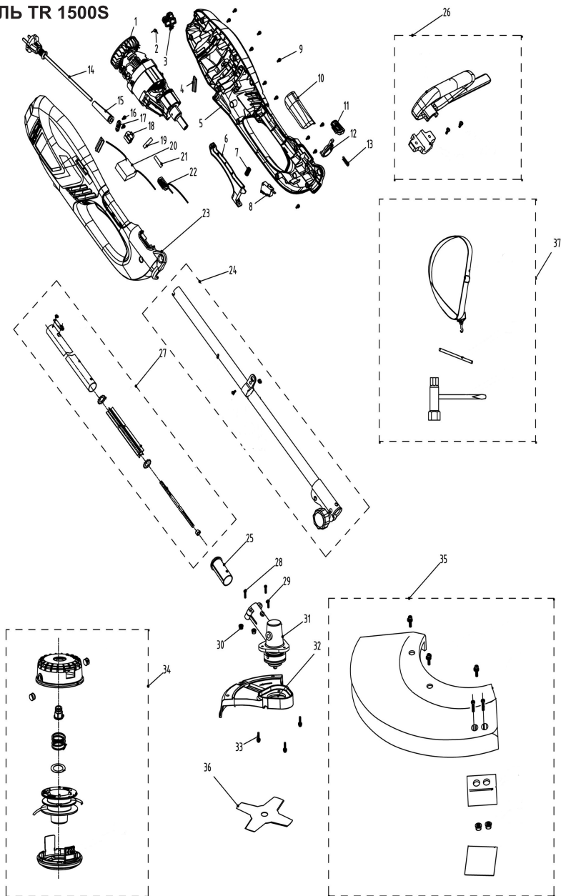
Рис. 6. Схема частей
