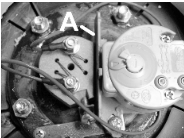
Пластиковый разделитель/А. Пластиковый разделитель
