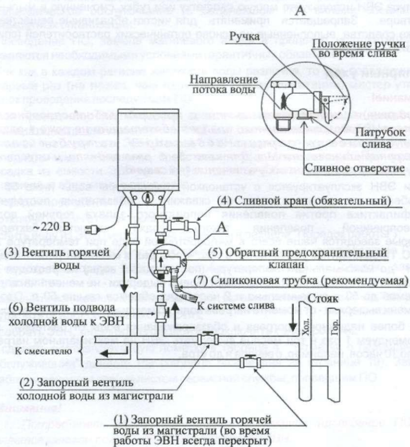
Рисунок 4 - Схема подключения к водопроводной сети
