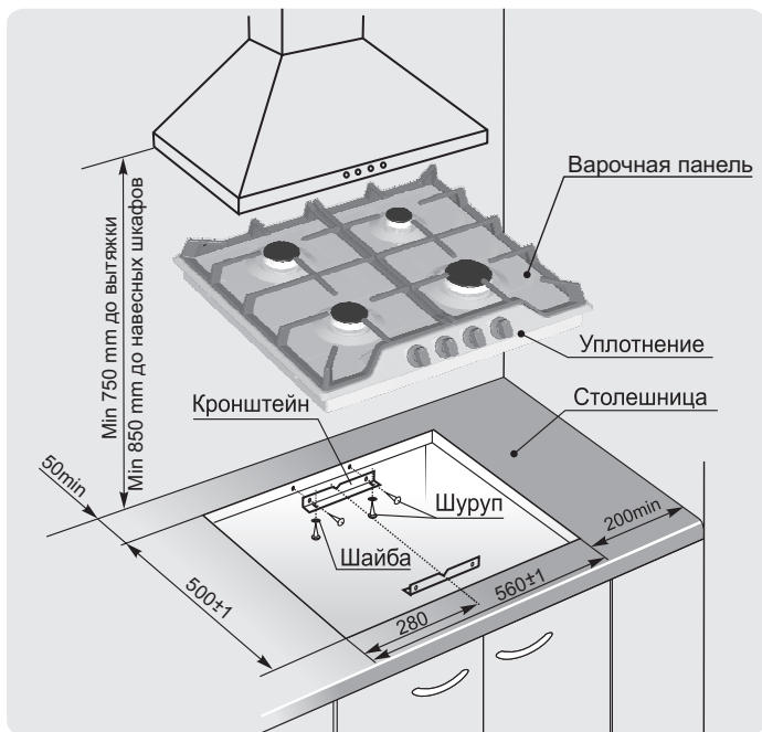
Рис. 3 МОДЕЛЬ ПВГ 1212; -01
