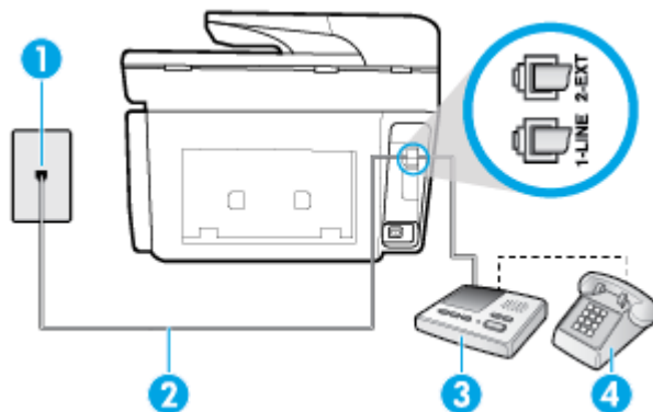
Рисунок 5-11 Вид принтера сзади
