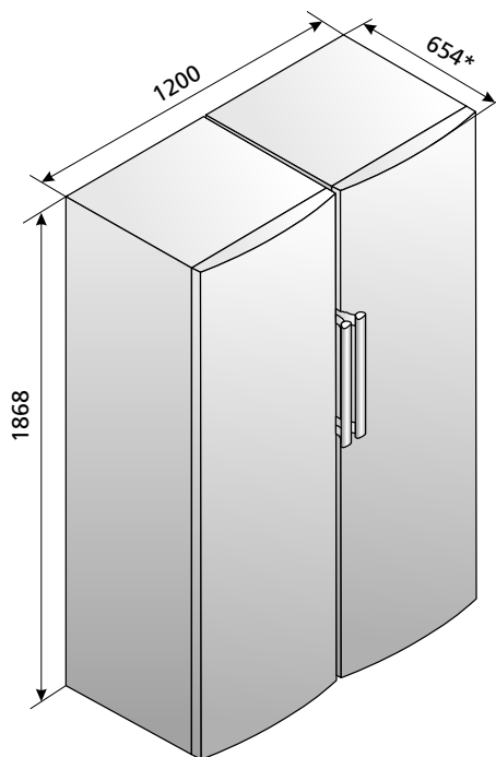
Рисунок 9 – Габаритні розміри комбінації Side by side
