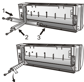
Возможные направления прокладки трубопровода
