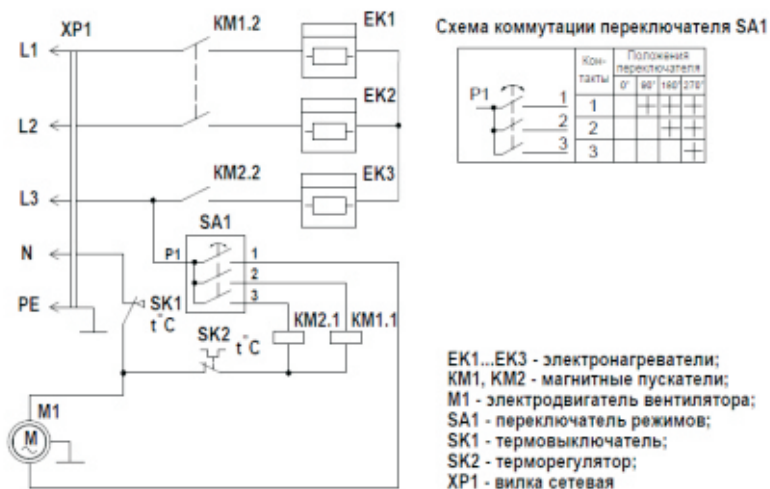
Рис.1 Схема электрическая
