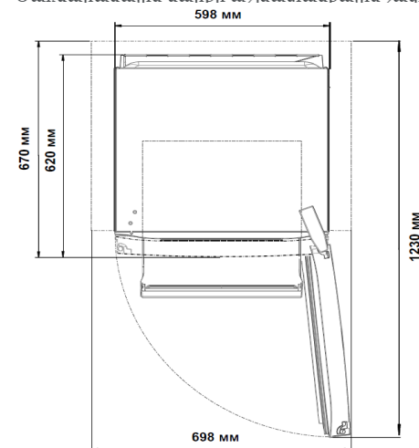
Սառնարանահին սառնի աշխատանքահին չափերը
