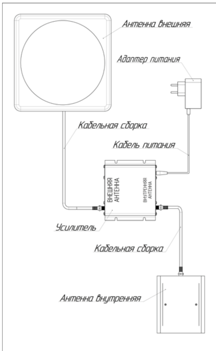
Рисунок 6. Схема подключения комплекта
