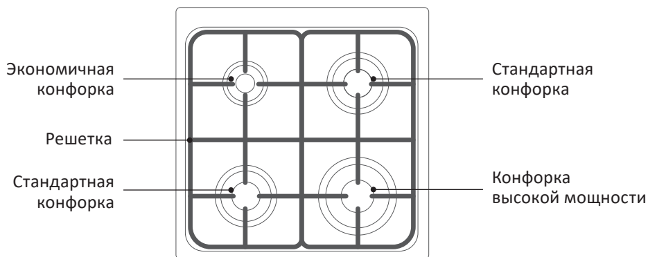
Расположение конфорок в модели M16-1
