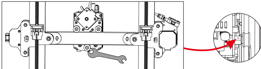
Печатающая головка
