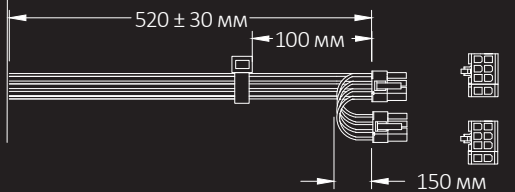
Разъем PCI Express (6 + 2)
