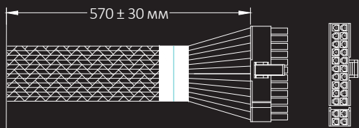
Разъем материнской платы
