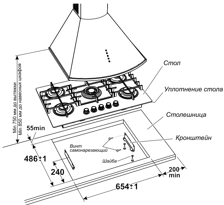
Рис. 7 МОДЕЛЬ СН2340
