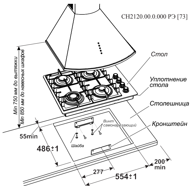
Рис. 6 МОДЕЛЬ СВН2230; -01
