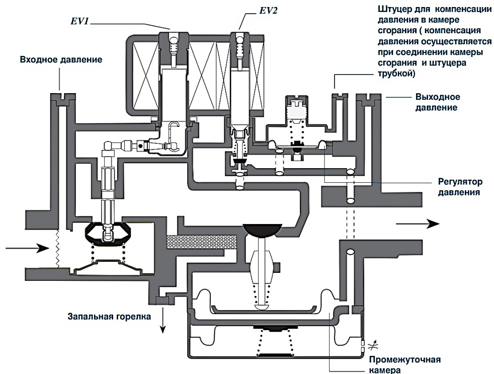
Рисунок 4б – Конструкция клапанов SIT 840 SIGMA и ERCO EBR2006N.
