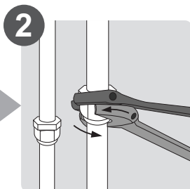
2 Присоедините трубы хладагента
