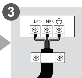
3 Подсоедините кабели
