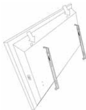
Bild 8. Befestigung des oberen Hakens, Hinteransicht
