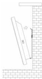
Obrázek 7. Připevnění horního háku na konvektor
