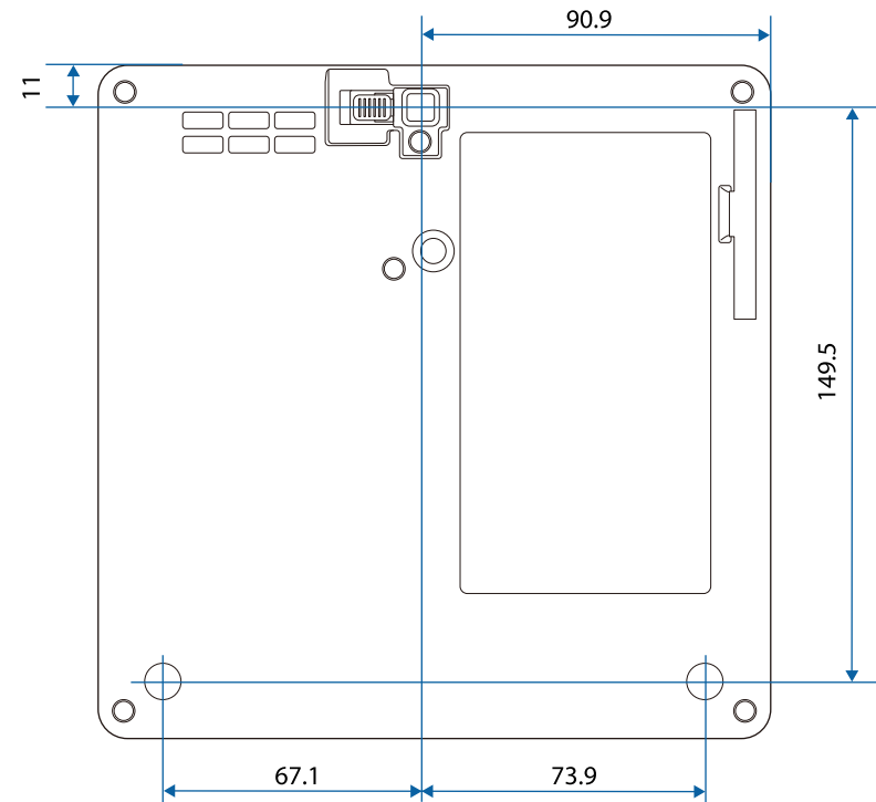
2 Расстояние от центра объектива до точки крепления кронштейна подвески
