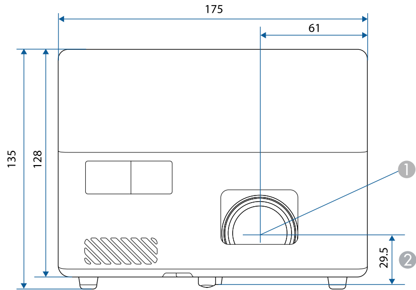
1 Центр объектива
