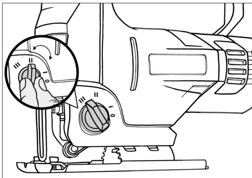
Рис. 7. Регулировка маятникового хода на модели Л-4350
