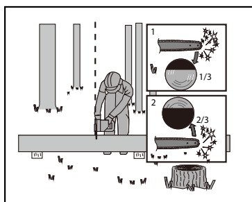
на месте верхнего запила. (См. рис. 5) Рис. 5
