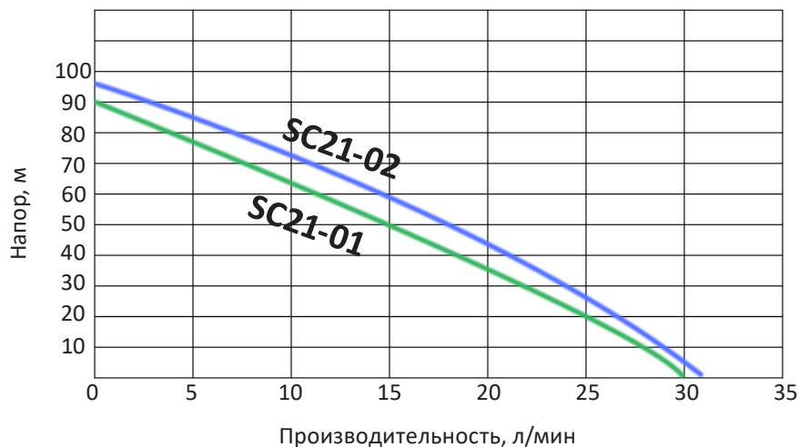
График расходно-напорных характеристик
