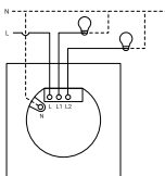
Схема подключения с нейтралью
