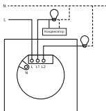
Схема подключения без нейтрали
