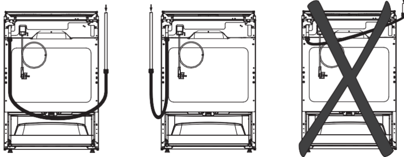
Иілгіш қосқышты қосу
