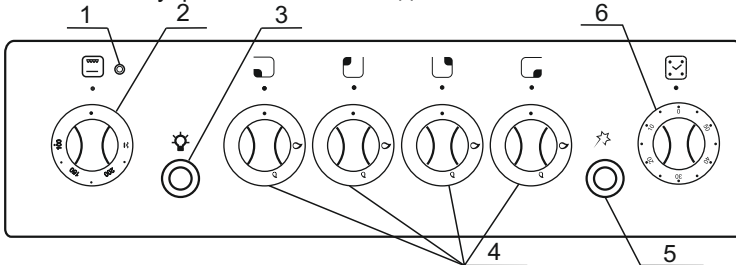
Панель управления плиты модели 506040.20гэ
