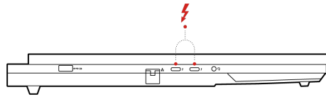
Рис. 4. Два многоцелевых разъема USB Type-C расположены на левой стороне ПК
