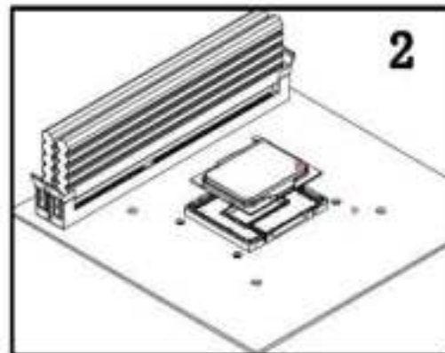
2. 将CPU按三角方向对齐安装
