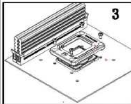
3. 安装BCF，用原配螺丝对称拧紧
