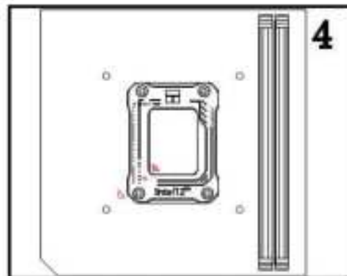
4. 注意安装方向，三角图形对齐
