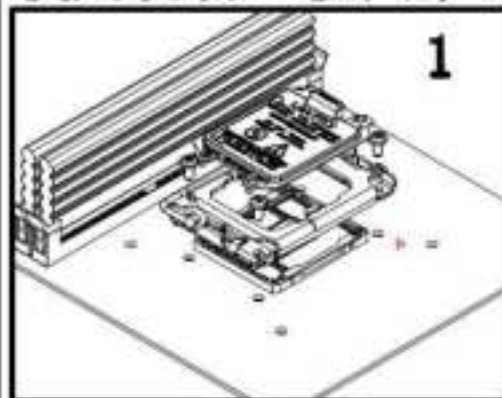
1. 用附赠螺丝刀拆除原装支架
