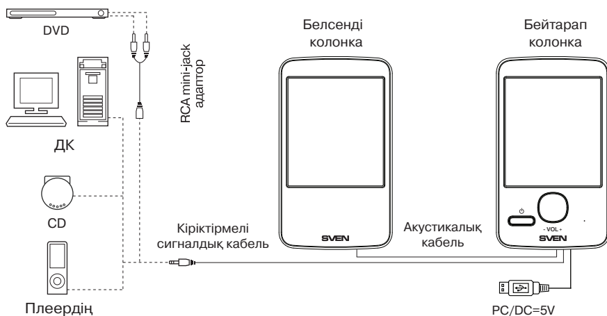
2-сурет. Қосу схемасы
