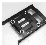
SSD-ді бұрандалармен жылжымаларға бекітіңіз
