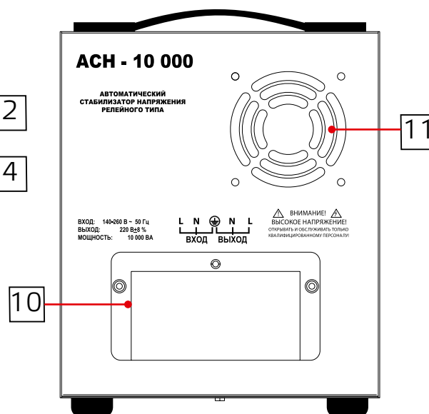
Задняя панель
