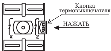
Рисунок 3 - Лицевая панель термовыключателя в моделях 3W30V1, 3W40V1, 3W50V1, 3W60V1
