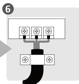
6 Электрлік сымдарды жалғаңыз
