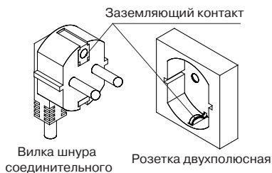
Рисунок 1 — Заземление плиты
