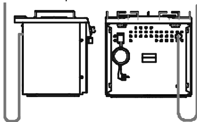
Рисунок 6 — Схема подсоединения газовых коммуникаций к плите
