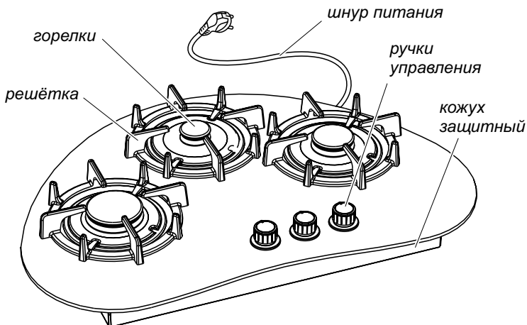
Рис. 1 МОДЕЛЬ CH2120
