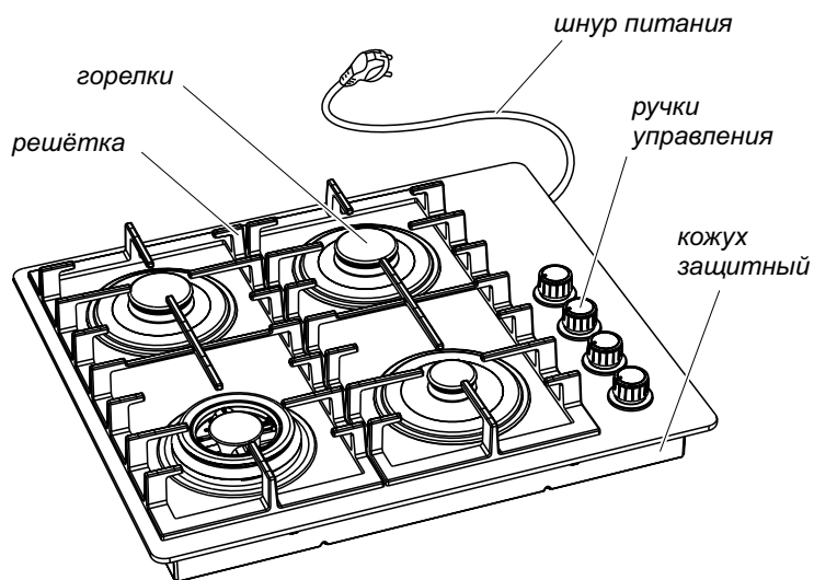
Рис. 2 МОДЕЛЬ CHN2230; -01
